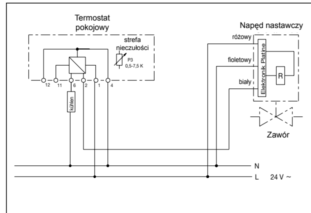
Schemat podłączenia
