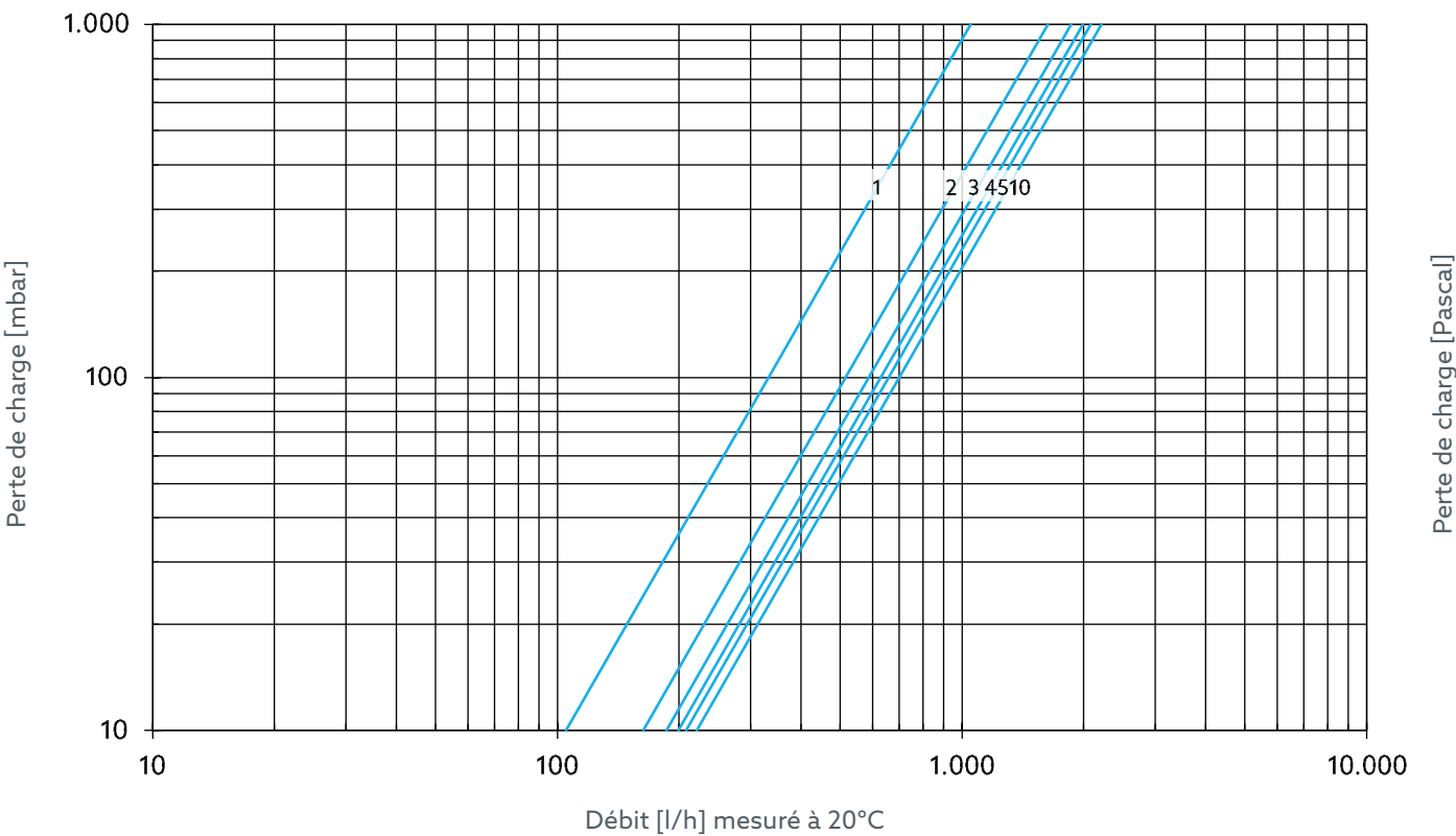
Fig. 16: Préréglage du débit DN 20
