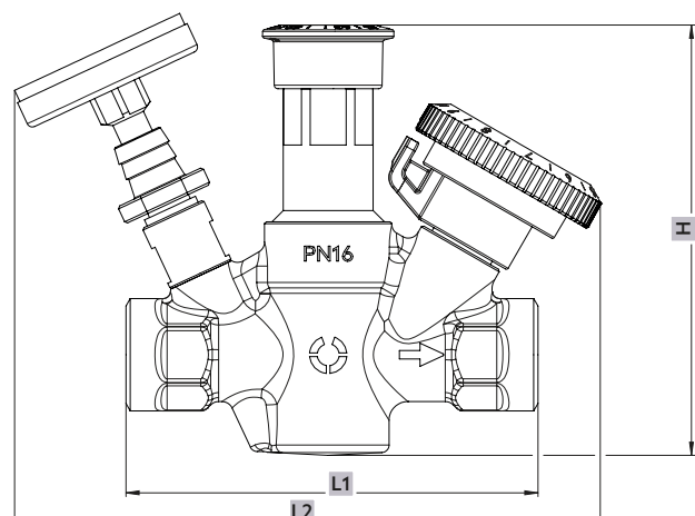
Afb. 2: Afmetingen lateraal
