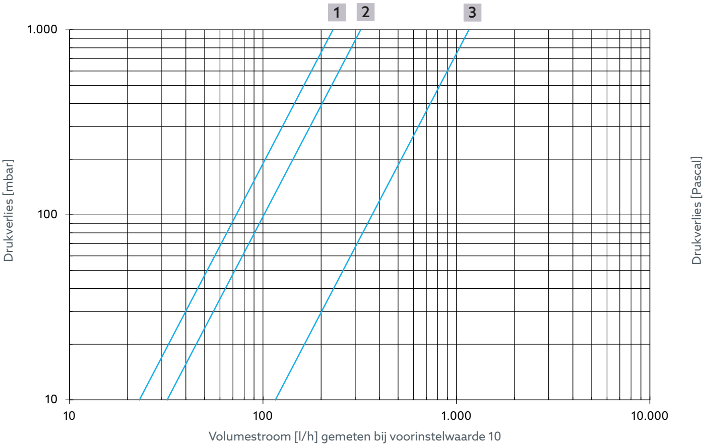
Afb. 18: Volumestroom Thermische regeling voor artikelnummers 4202553 en 4202753
