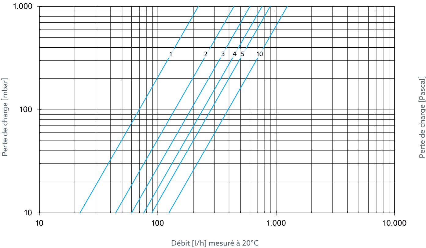
Fig. 15: Préréglage du débit DN 15
