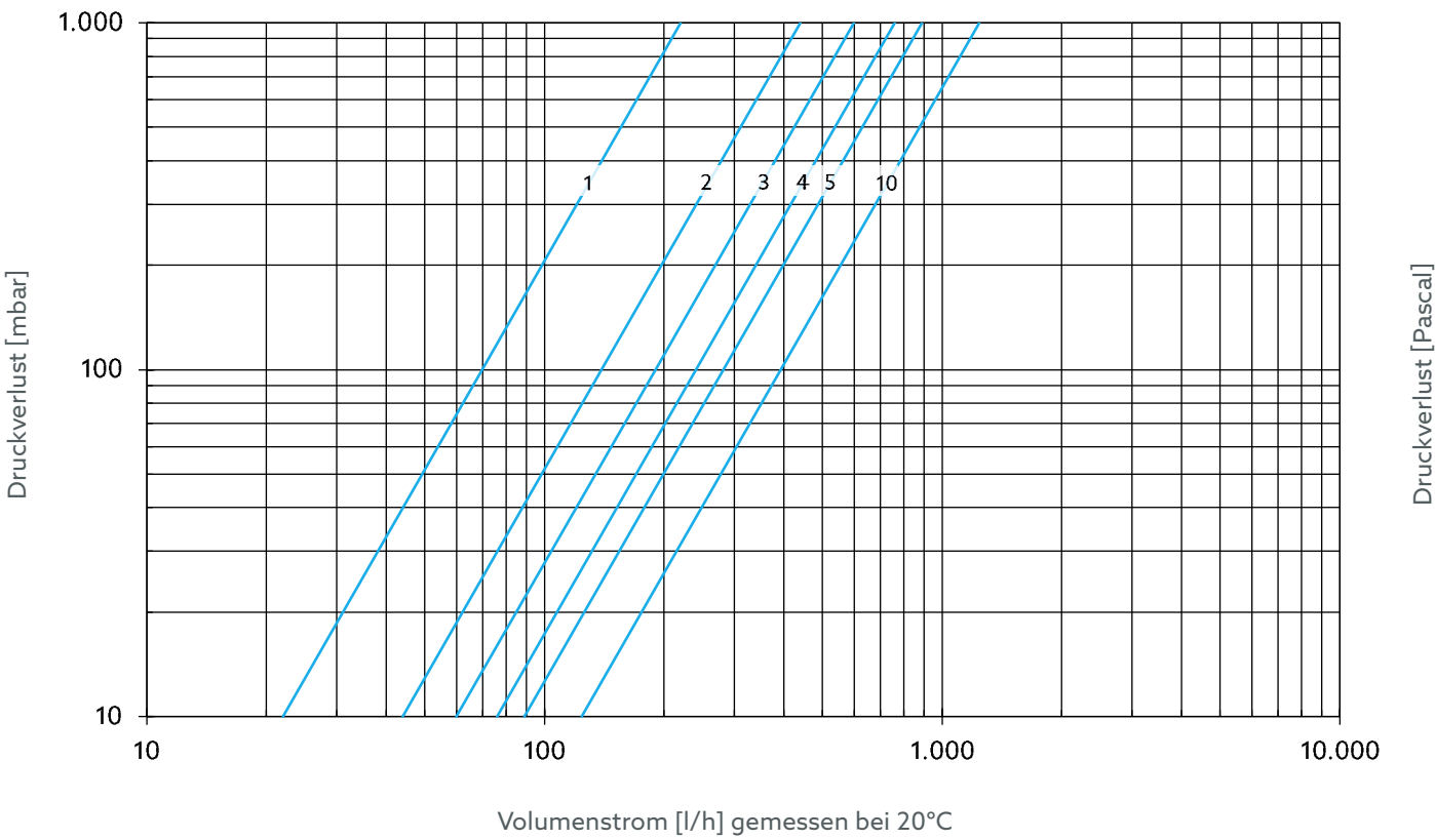
Abb. 15: Volumenstromvoreinstellung DN 15
