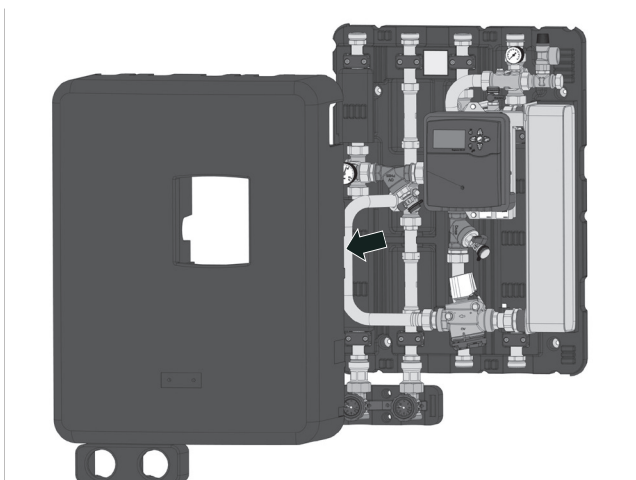
Abb. 26: Wärmedämmoberschalen entfernen
