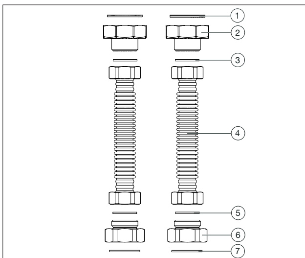
Abb. 29: Aufbau Verbindungsset
