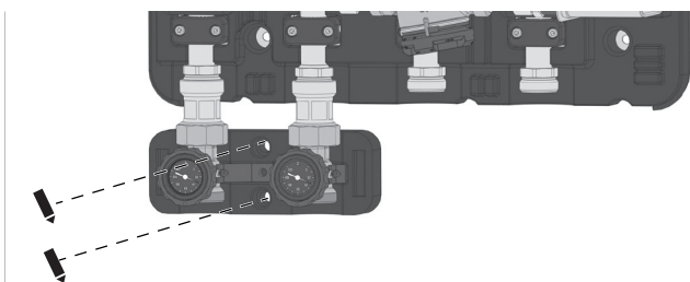
Abb. 27: Bohrlocher Befestigungsschrauben markieren
