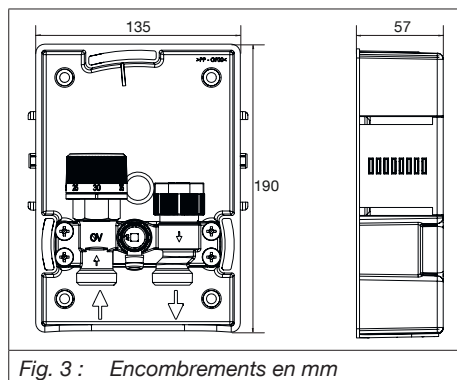
Fig. 3 : Encombresments en mm
