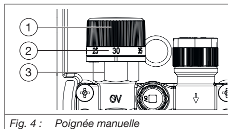
Fig. 4 : Poignée manuelle
