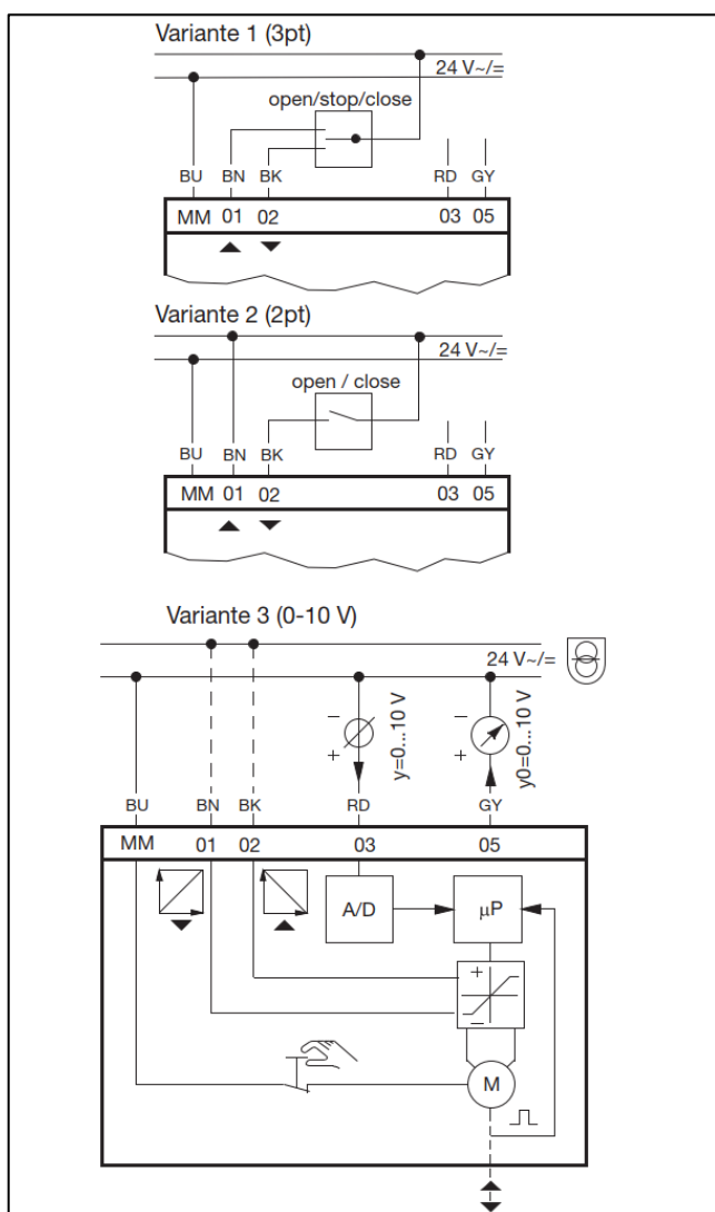
Schaltpläne Art.-Nr.: 1158011
