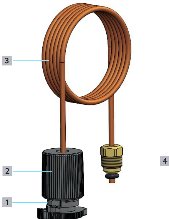
Abb. 4: Aufbau Impulsleitung
