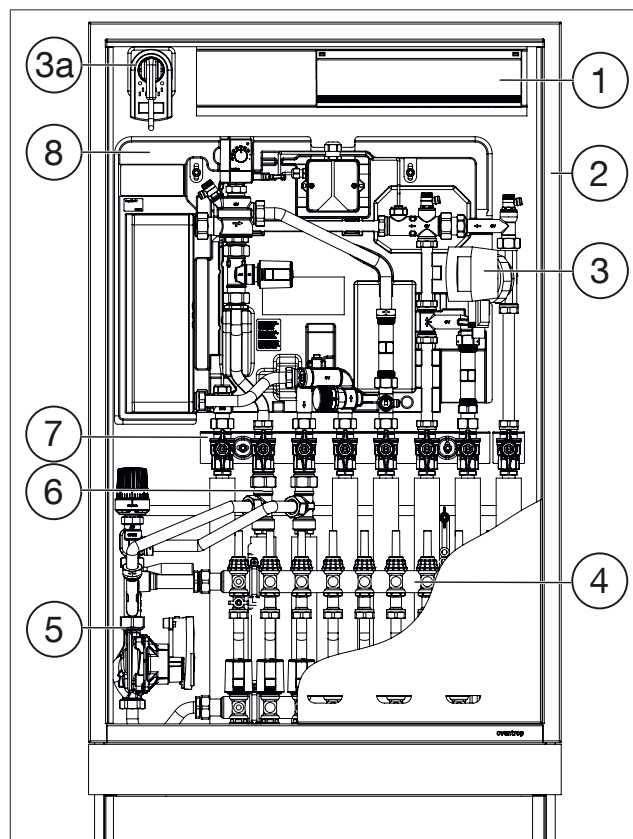
Fig. 3: Exemple d'installation
