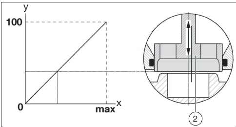
Abb. 5: Lineare Kennlinie der Reguliereinheit
