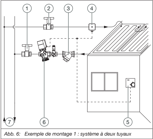
Abb. 6: Exemple de montage 1 : système à deux tuyaux
