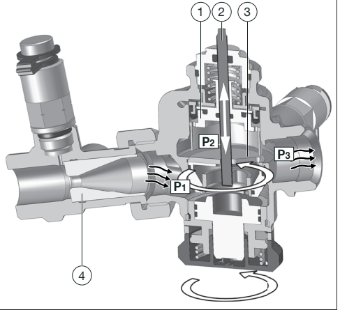
Abb. 2: „Cocon QTZ“ mit Messblende Querschnitt
