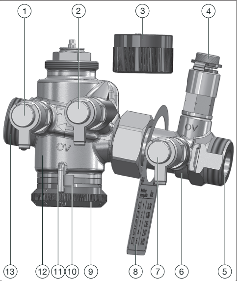
Abb. 1: „Cocon QTZ“ mit Messblende
