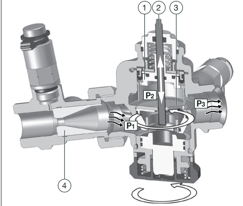
Abb. 2: « Cocon QTZ » avec diaphragme de mesure en coupe transversale
