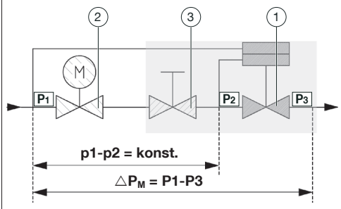
Abb. 3: „Cocon QTZ“ Funktionsschema
