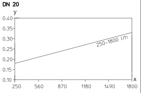
Abb. 16: Mindest-Differenzdrücke
