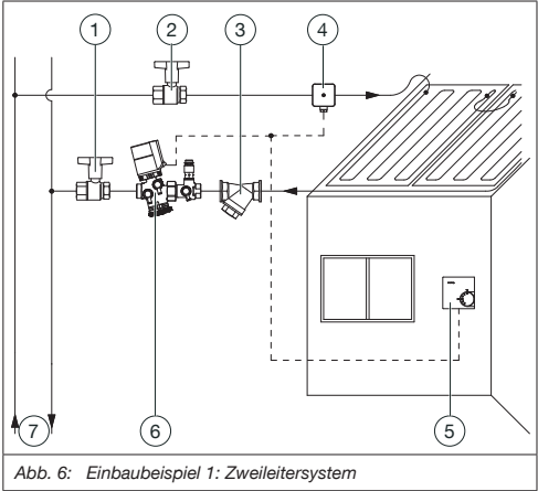
Abb. 6: Einbaubeispiel 1: Zweileitersystem
