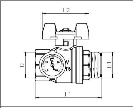
Abb. 5: Maße Kugelhahn
