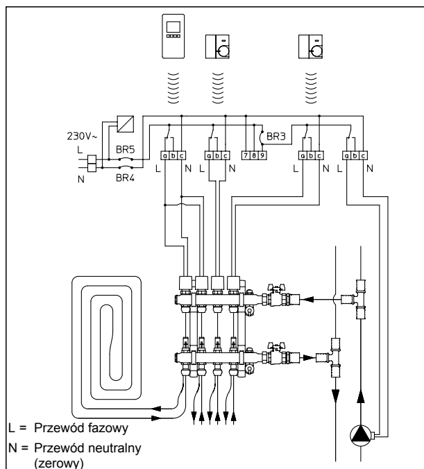
Przykład zastosowania 2. Schemat połączeń
