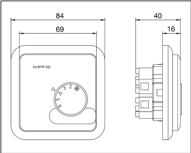
Encombrements du thermostat d'ambiance
