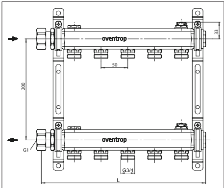
Abb. 2: Maße in mm (Frontansicht)
