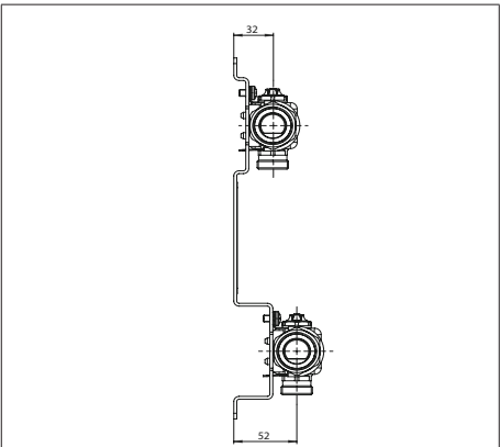
Fig. 3: Dimensions en mm (vue de côté)
