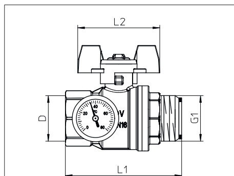
Fig. 4: Dimensions robinet à tournant sphérique en mm
