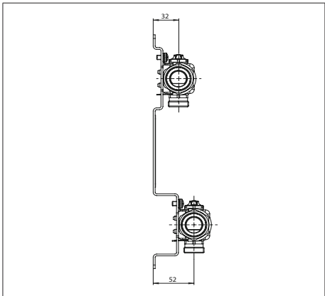
Abb. 3: Maße in mm (Seitenansicht)
