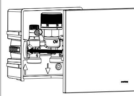
Abb. 7: Abdeckung aufsetzen
