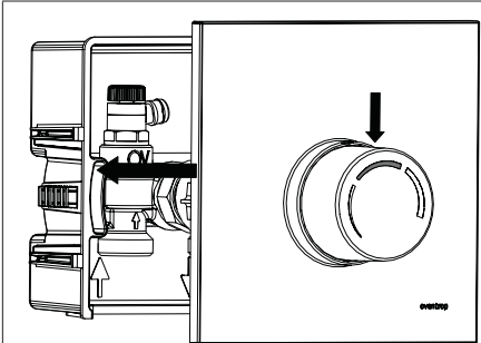
Abb. 6: Abdeckung mit Handrad aufsetzen
