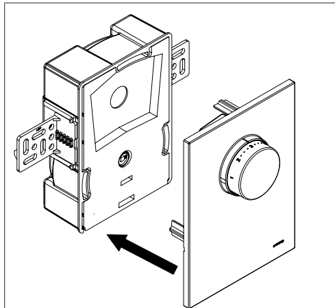
Fig. 9: Montage du capot avec poignée manuelle
