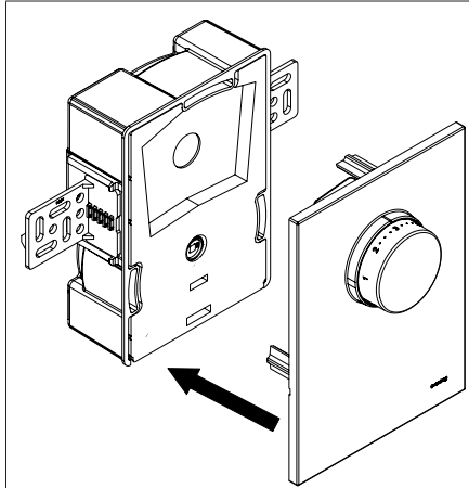
Abb. 9: Abdeckung mit Handrad aufsetzen
