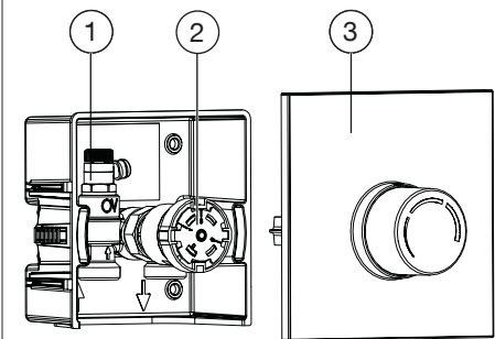
Abb. 1: Aufbau „Unibox RTL vario“
