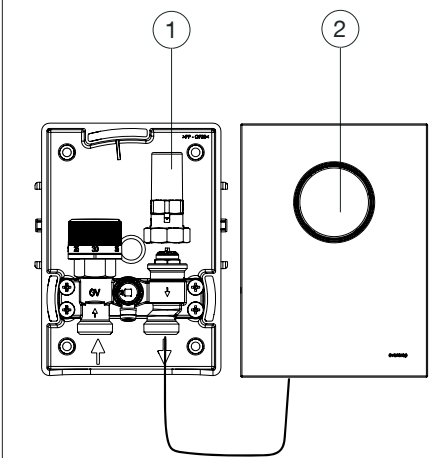
Abb. 8: Thermostat mit Fernversteller montieren
