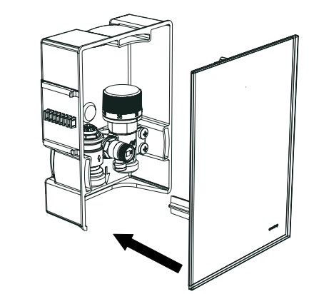
Abb. 10: Abdeckung aufsetzen
