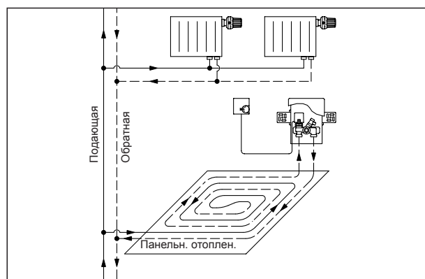
Схема монтажа „Unibox vario“ с термостатом и приводом
