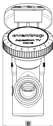
Obr. 3: Čelné rozmery
