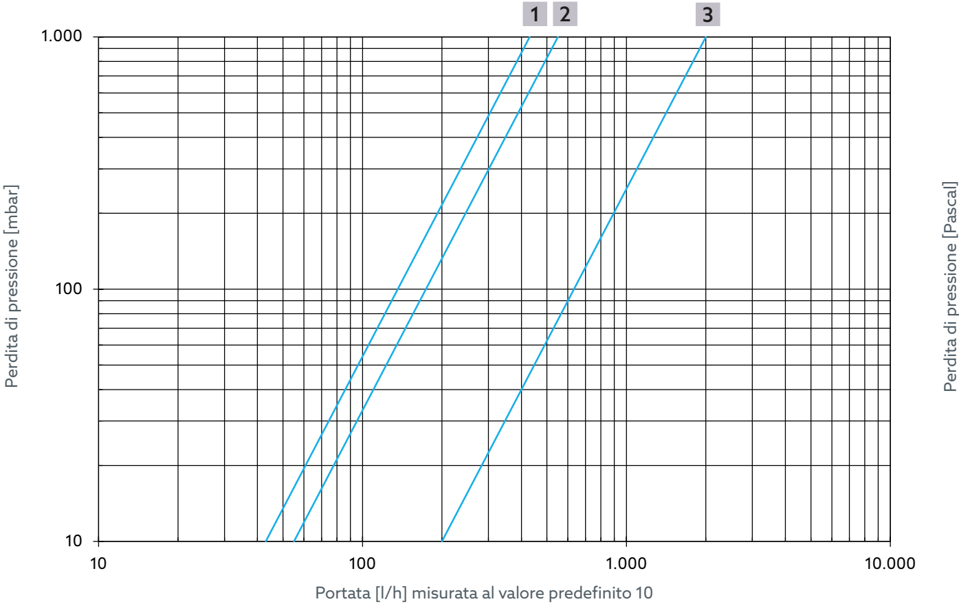
Fig. 20 - Portata regolazione termica dei codici articolo 4202554 e 4202754
