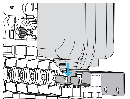
Fig. 12: Position de montage du support inférieur pour le vase d'expansion à membrane dans le coffret
