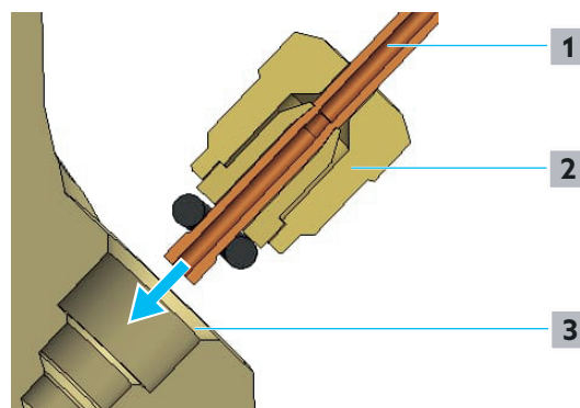
7. Az impulzuscső csatlakoztatása a HydroControl D-re
