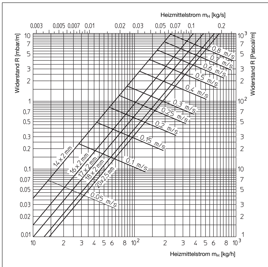
Diagramm 3: Druckverlustrdiagramm für Oventrop-Rohre
