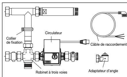
Fig. 5.1 Vue d'ensemble «Regufloor HC»
