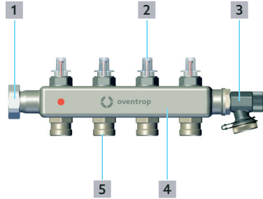
Fig. 2: Construction du distributeur pour l'aller du distributeur/collecteur pour circuits de chauffage Multidis SFQ
