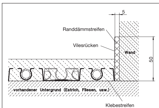
Maße Randdämmstreifen
