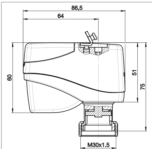
Abb. 2: Seitenansicht
