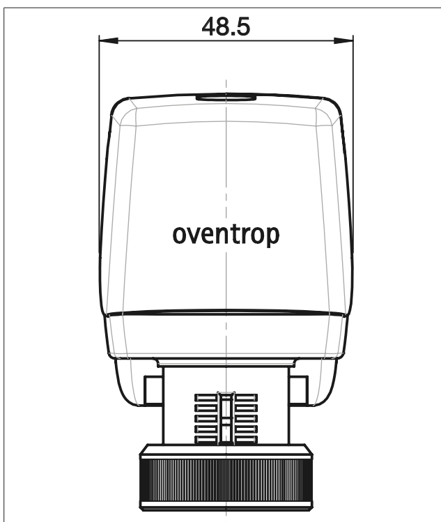
Abb. 3: Vorderansicht
