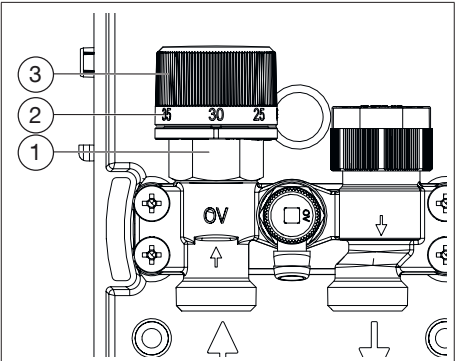
Fig. 4: Poignée manuelle
