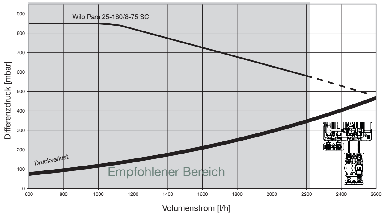
Abb. 5: Druckverlust Sekundärkreis Regudis H-H
