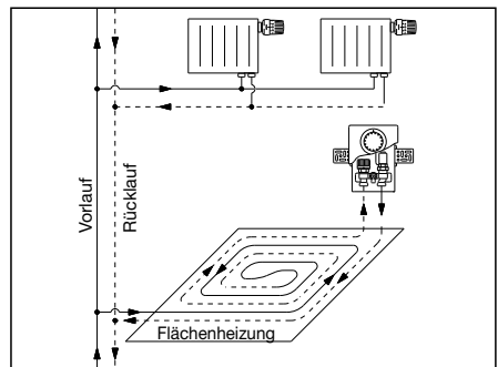
Einbauskeizze
