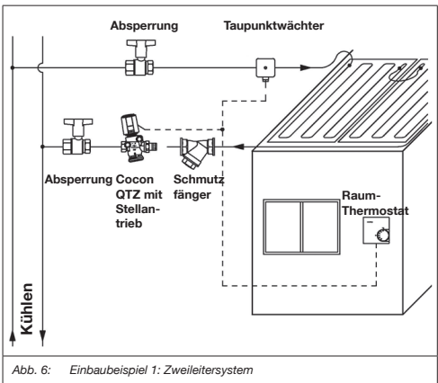
Abb. 6: Einbaubeispiel 1: Zweileitersystem
