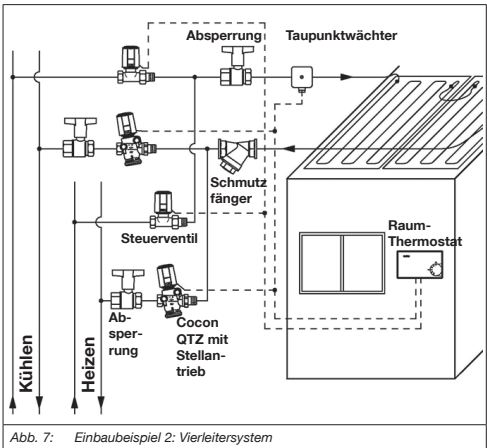
Abb. 7: Einbaubeispiel 2: Dreileitersystem
