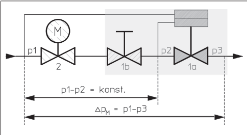
Abb. 3: Funktionsprinzip „Cocon QTZ“, PN25
