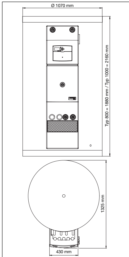
Abb. 2 Abmessungen
