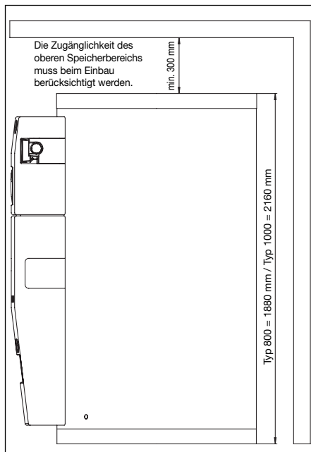
Abb. 4 Einbaumaße
