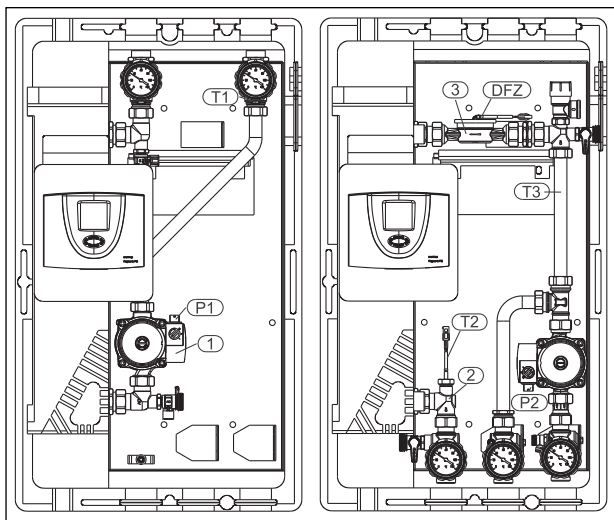
Abb. 1: „Regumaq XZ-30“ Primär- und Sekundärkreis
