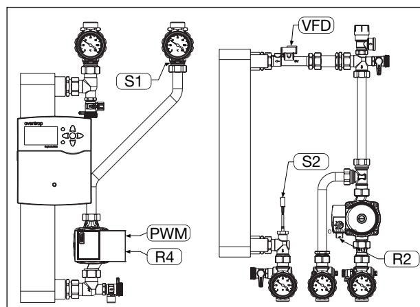
Abb. 3: „Regumaq XZ-30-B“ Primär- und Sekundärkreis
