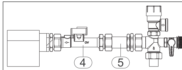
Abb. 2: Montage Vortex Volumenstromsensor
