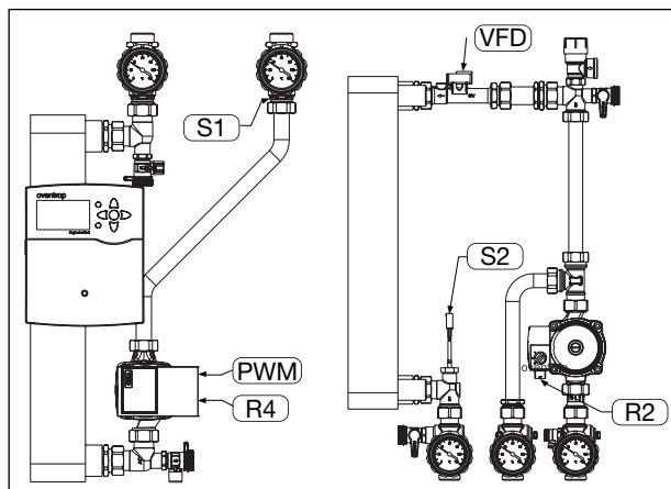
Fig. 3: «Regumaq XZ-30-B» Circuit primaire et secondaire
