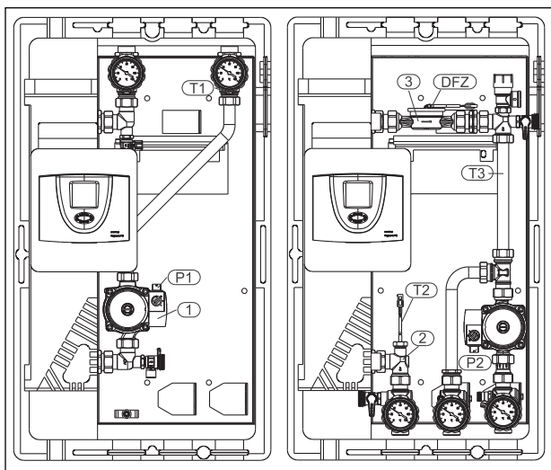
Fig. 1: «Regumaq XZ-30» Circuit primaire et secondaire
