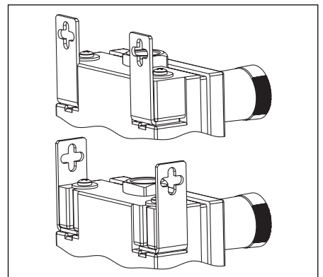
Abb. 6.1 Winkelmontage hinten (oben) und seitlich (unten)
