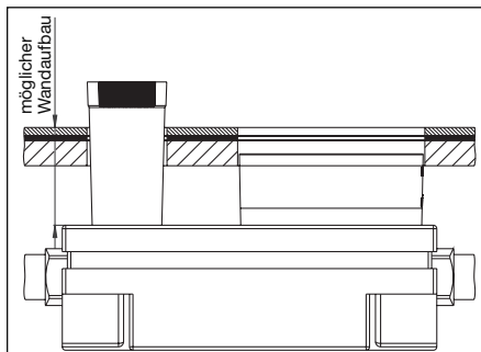
Abb. 4.2 Beispiel Wandaufbau
