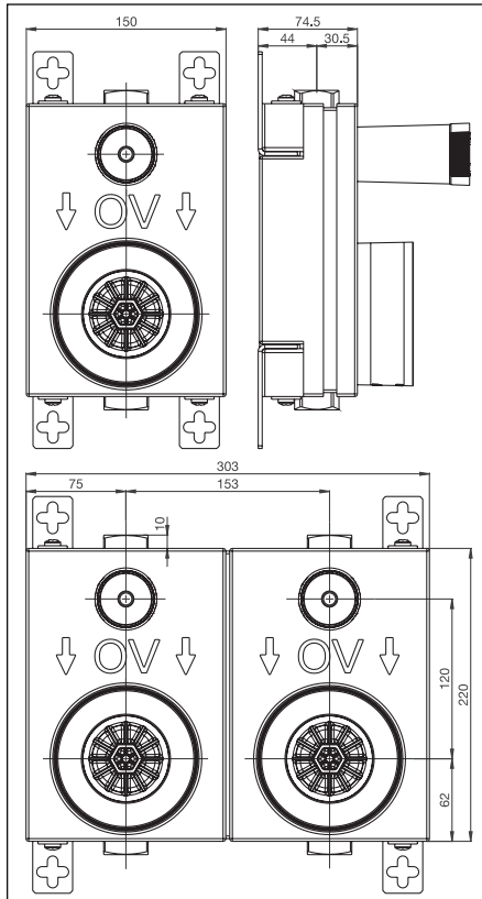
Abb. 4.1 Abmessungen und Einbaumaße
