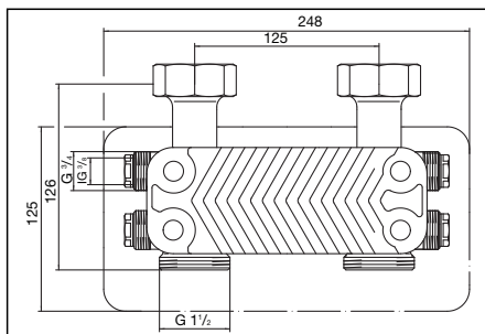
„Regumat“ Wärmeübertrager
