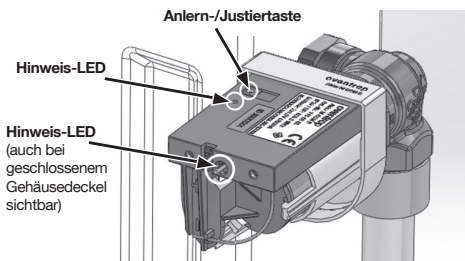
Abb. 18: Hinweis-LEDs am Funk-Stellantrieb „mote 320“ nach „Justierfahrt“
