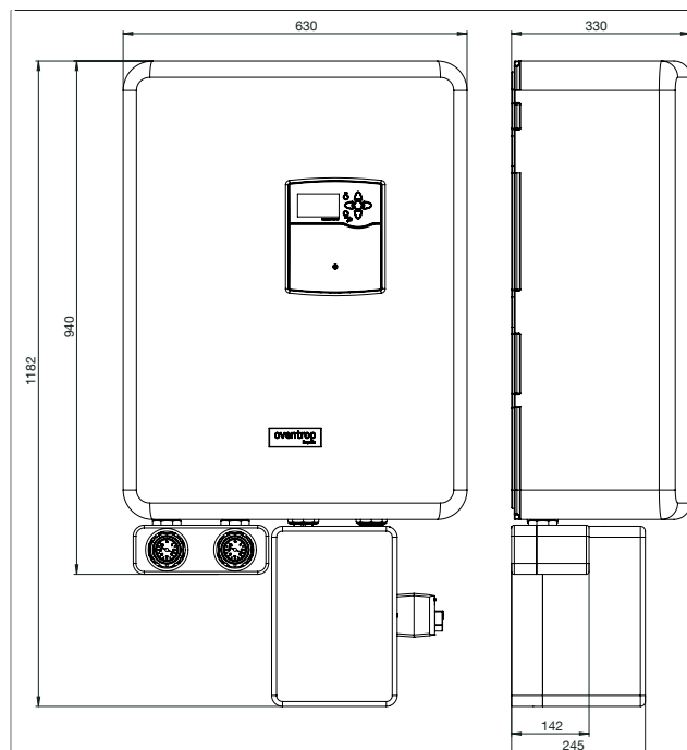
Abb. 3: Abmessungen in mm
