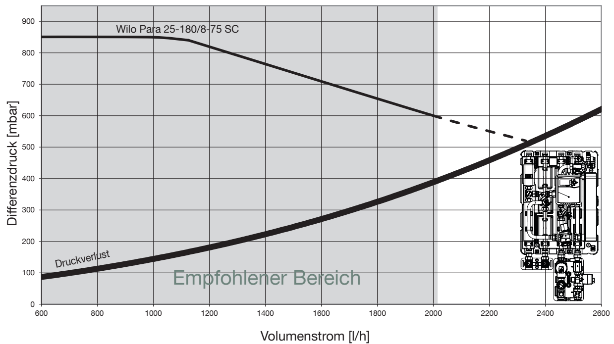
Abb. 5: Druckverlust Sekundärkreis Regudis H-MT
