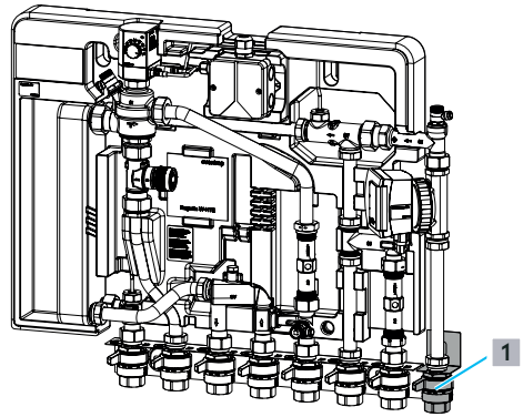
Abb. 1: Einbauort
