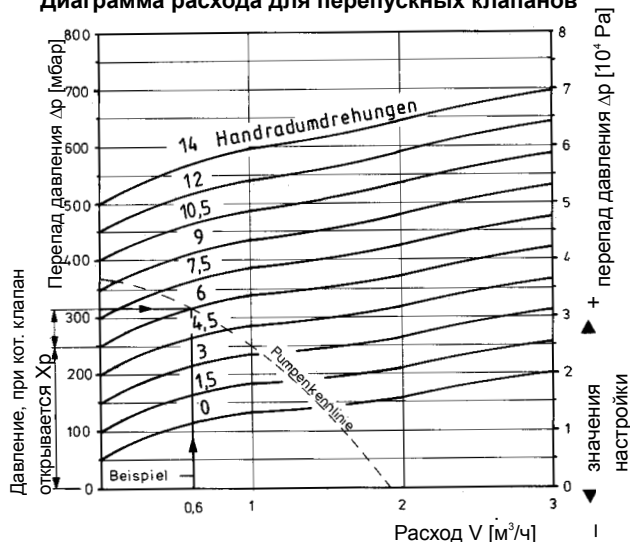
Диаграмма расхода для перепускных клапанов
