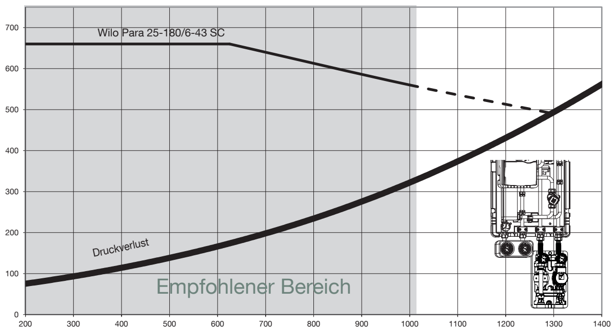
Abb. 5: Druckverlust Sekundärkreis Regudis H-H
