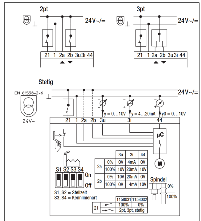
Schaltpläne, Art.-Nr. 1158031/32
