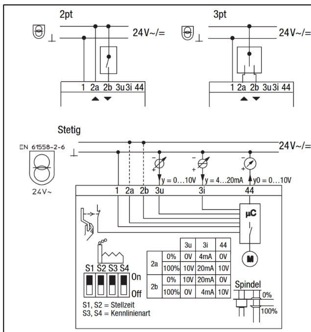
Schaltpläne, Art.-Nr. 1158030
