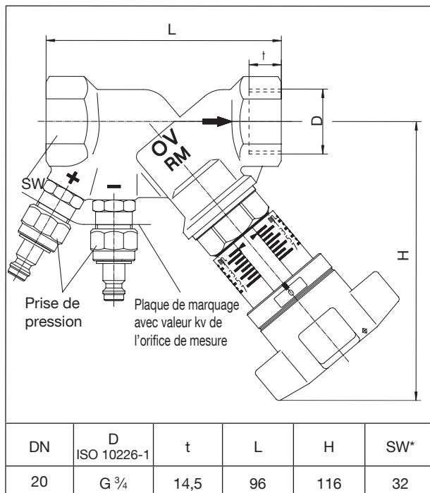
« Hydrocontrol STR » avec filetage femelle selon EN 10226 des deux côtés
