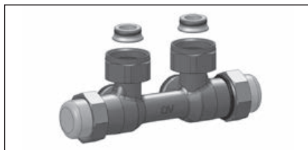
Abb. 2 Anschlussarmatur „Multiflex FQ“, Eck, Linksan- schluss, G ¾ ÜM x G ¾ AG
