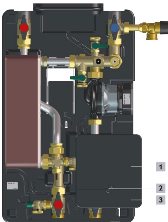
Abb. 29: Regler öffnen
