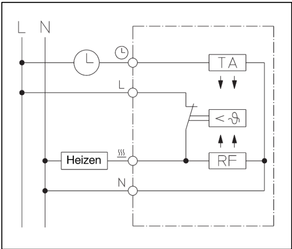
Schaltplan
