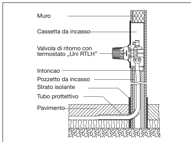
„Unibox RTL“, prof. 57 mm
