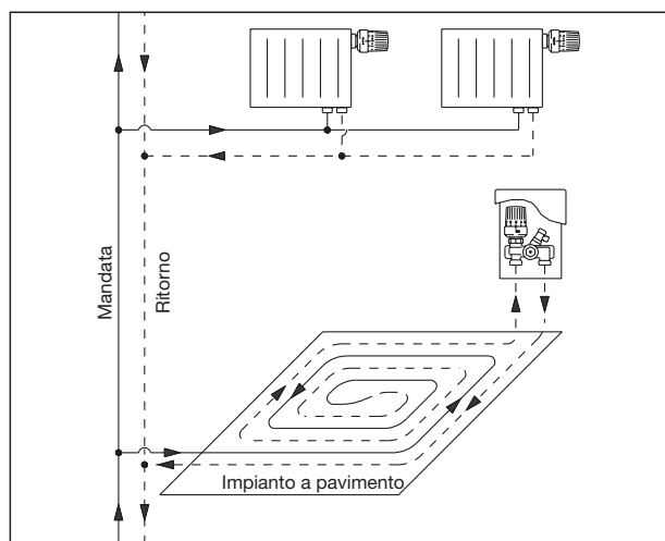
Schizzo di montaggio delle regolazione temp. ambiente e limitazione della temperatura in ritorno
