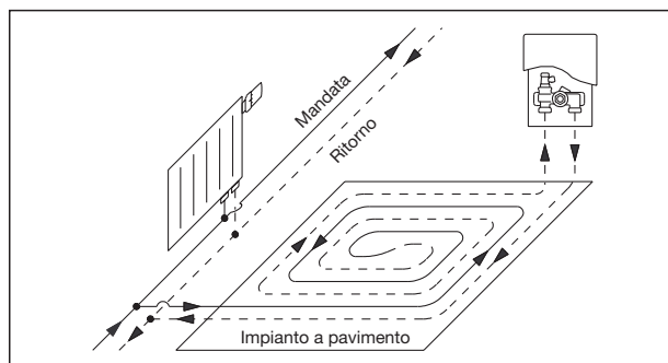
Schizzo di montaggio limitazione della temperatura di ritorno
