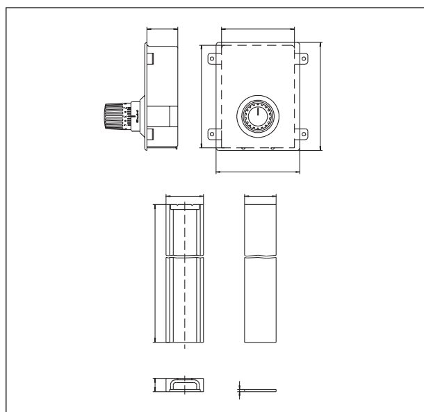
Dimensioni „Unibox“, prof. 57 mm e pozzetto da incasso
