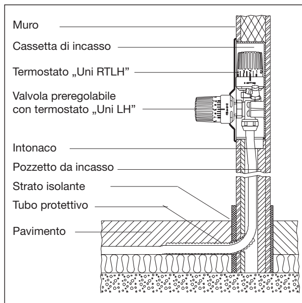
„Unibox plus”, prof. 57 mm
