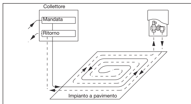
Schizzo di montaggio regolazione della temp. per ambiente
