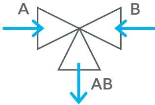
Einsatz als Mischventil: Volumenströme A und B werden hubabhängig auf AB vermischt
