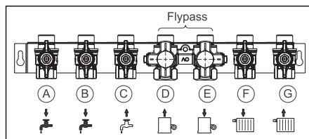
Abb. 5.1 Anschlusskennzeichnung
