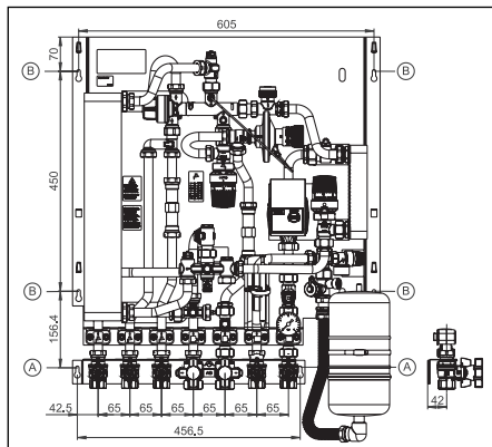
Abb. 6.1 Anschlussschema Kugelhahnanschlussleiste
