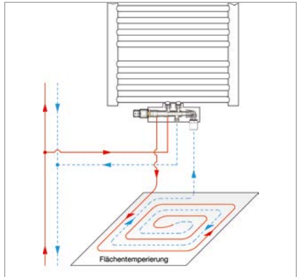
System-Darstellung „Multiblock T-RTL“ mit Flächenheizung
