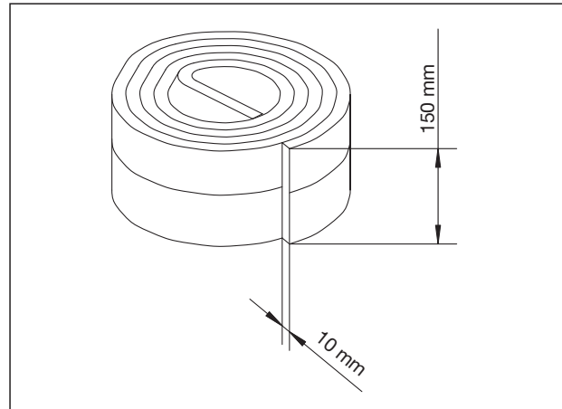
Maße Randdämmstreifen
