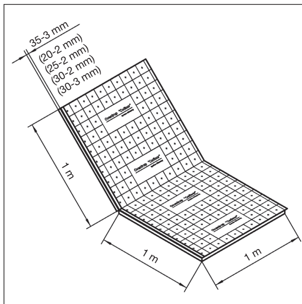
Maße Faltplatte
