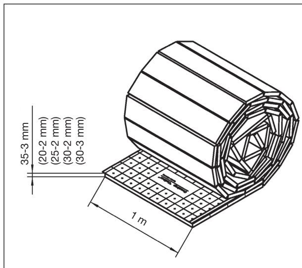
Maße Dämmrolle
