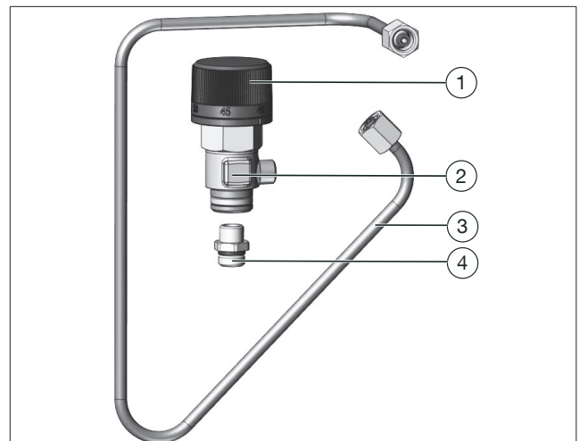
Abb. 1: Aufbau
