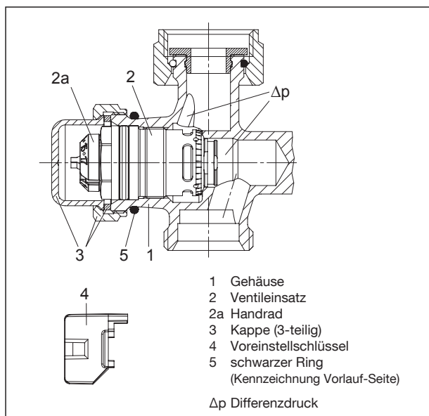
Aufbau Durchflussregler
