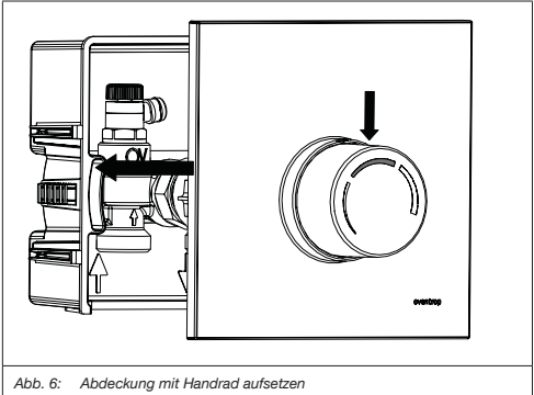
Abb. 6: Abdeckung mit Handrad aufsetzen
