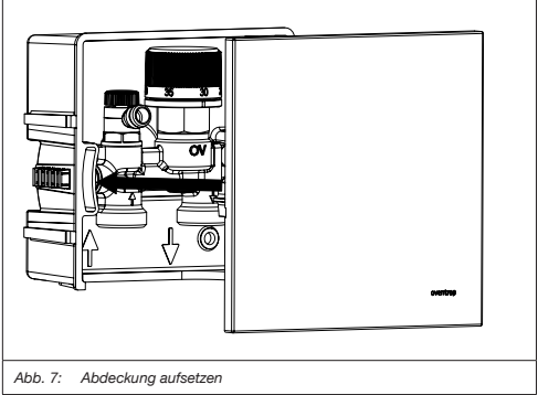
Abb. 7: Abdeckung aufsetzen
