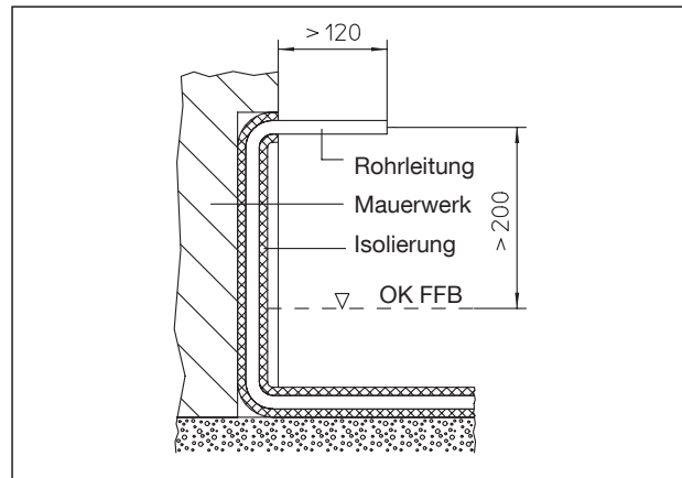
Schnitt, Heizkreisanschluss
