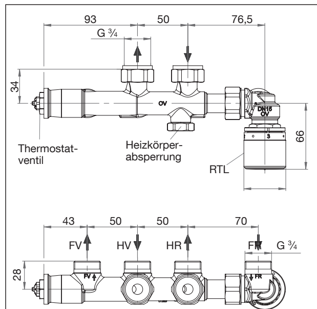
Abmessungen Armatur
