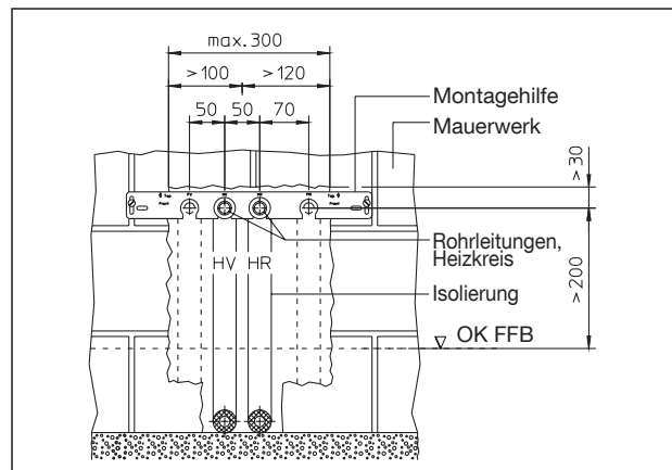
Wandansicht, Heizkreisanschluss
