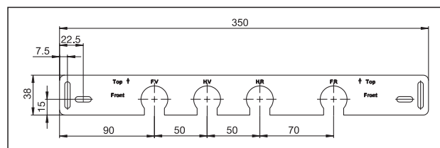
Abmessungen Montagehilfe
