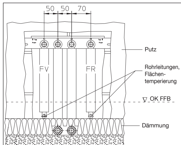
Wandansicht, Flächentemperierungskreisanschluss
