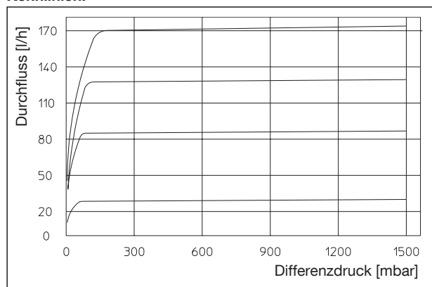
Thermostatventilkennlinien bei verschiedenen Handrad-Voreinstellungen im Volllastbetrieb
