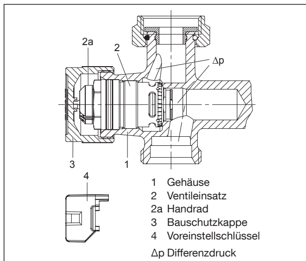
Aufbau Thermostatventil (Prinzipdarstellung)
