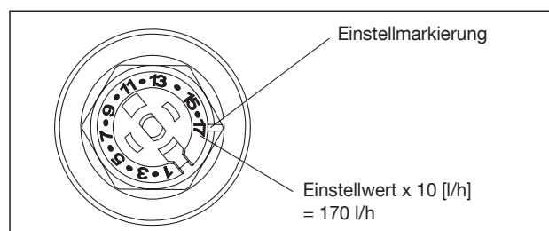
Durchflusseinstellung Thermostatventil
