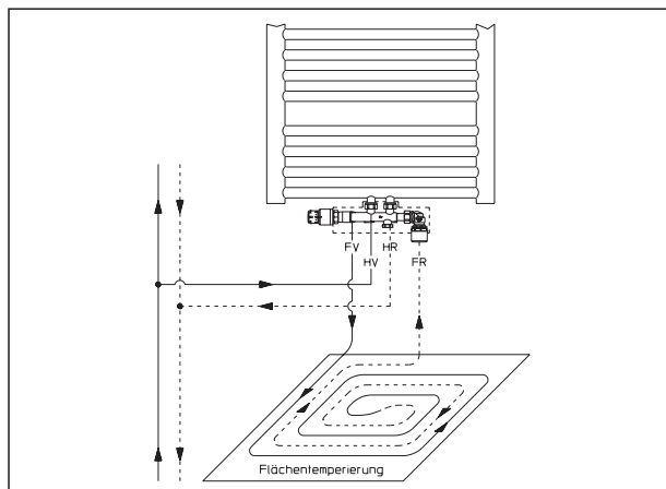
Systemdarstellung
