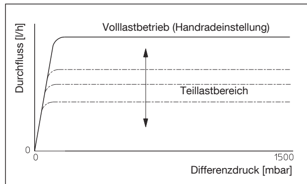
Thermostatventilkennlinien im Teillastbetrieb
