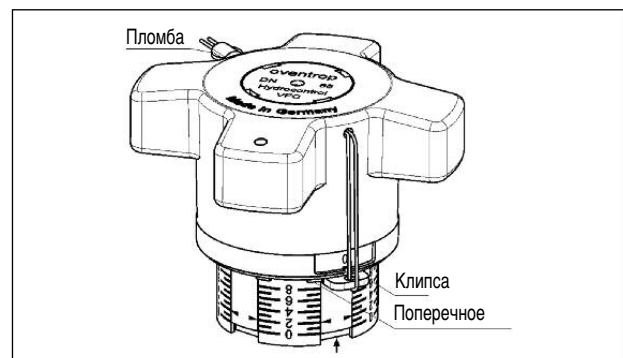
Рис. 7.2 Блокировка маховика
