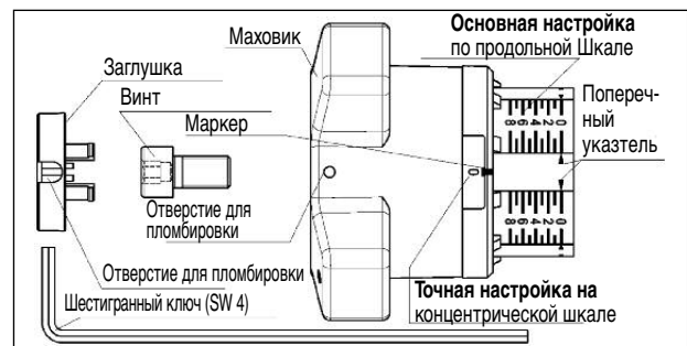
Рис. 7.1 Настройка
